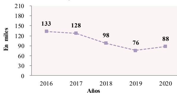
DESEMPLEO EN AGOSTO No Ajustado Estacionalmente
